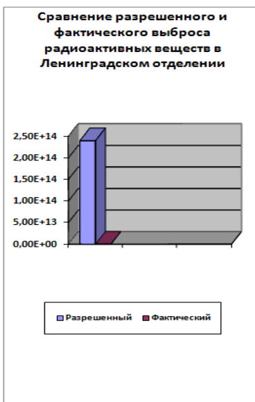
Рисунок 3 Сравнение разрешенного и фактического выброса радиоактивных веществ в Ленинградском отделении
